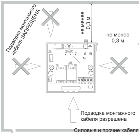
Рис.5. Установка базового блока.
