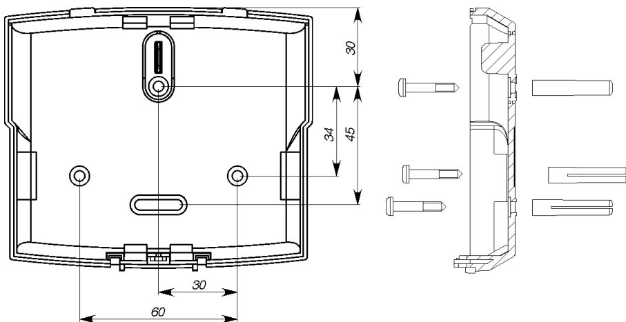
Рис.6. Разметка крепежных отверстий для клавиатуры M4064KP
