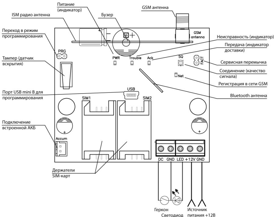
Рис. 7. Внешний вид платы прибора
