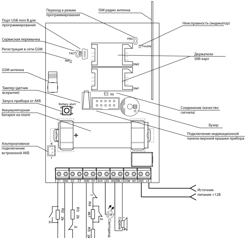
Рис. 6. Внешний вид платы прибора
