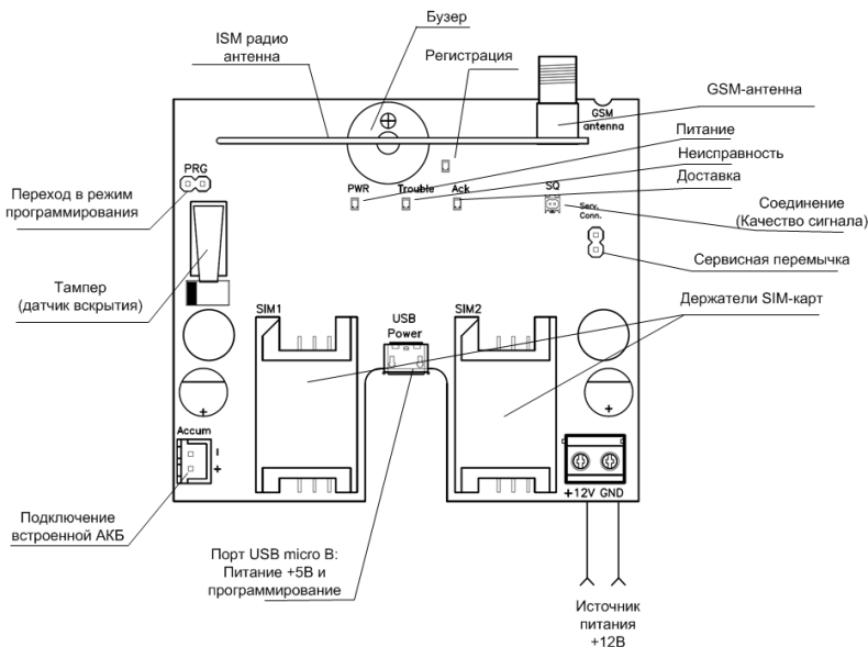
Рис. 7. Внешний вид платы прибора
