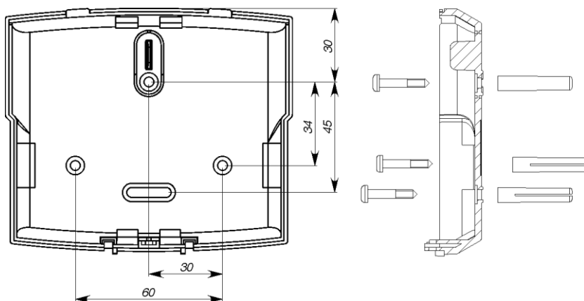
Рис.6б. Разметка крепежных отверстий для клавиатуры M4064KP
