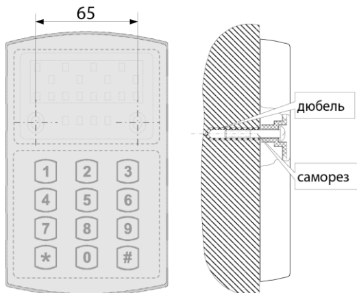
Рис.6а. Разметка крепежных отверстий для клавиатуры M8022KP
